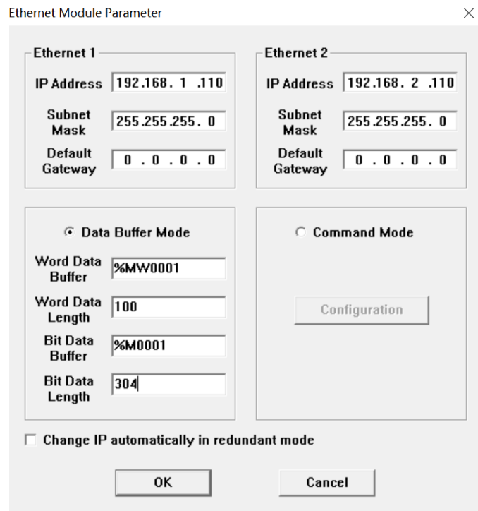
Рисунок 3.2 Настройки модуля CM 4000-0205
